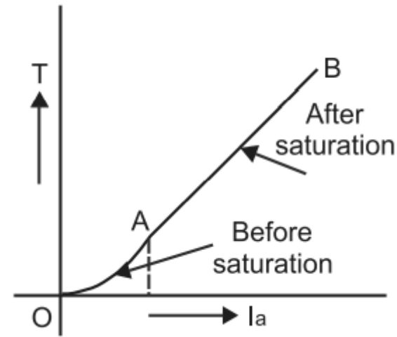
Fig. 3.11 T-I_a
