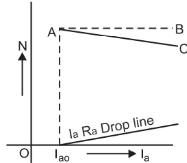
Fig. 3.7 N - I_a
